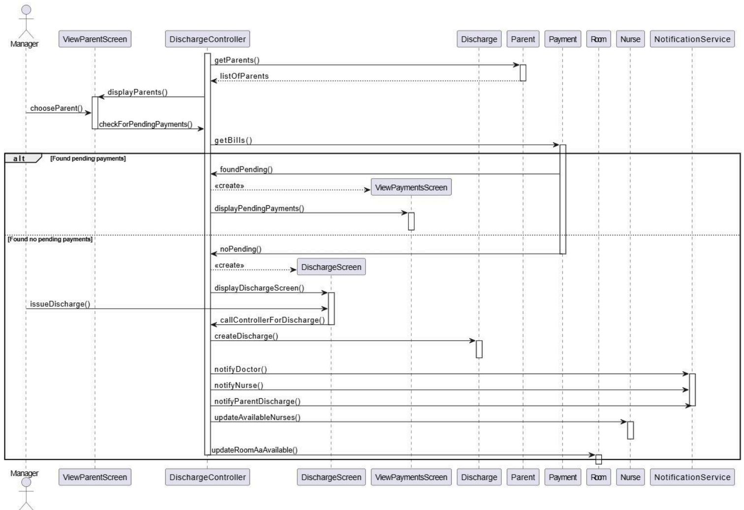
Sequence Diagram 6: Εκδοση εξιτηρίου
